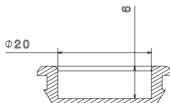
Section view A-A Scale: 2:1
